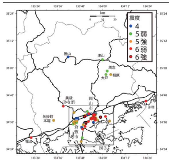
写真⑦ 安政南海地震(1854)の岡山県全体の震度分布図
