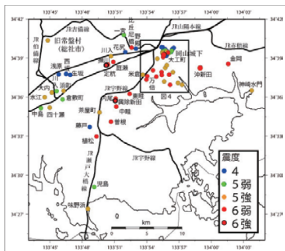
写真⑧ 安政南海地震の岡山市および倉敷市とその周辺の震度分布
