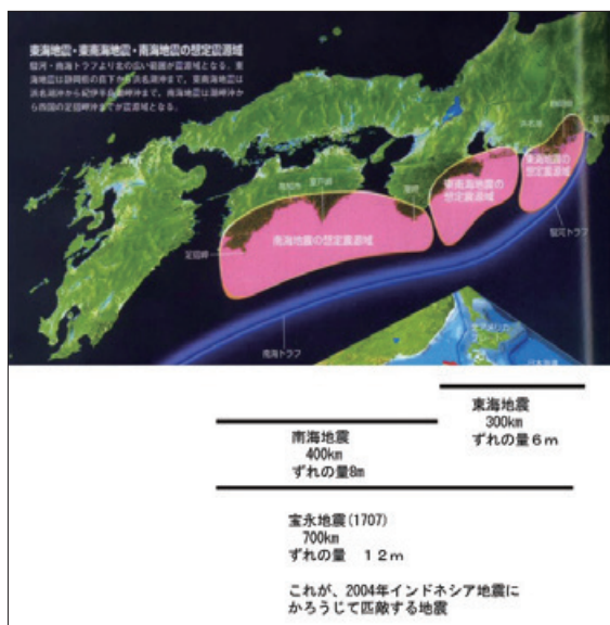
写真① 南海プレートと東海地震・南海地震の震源域
