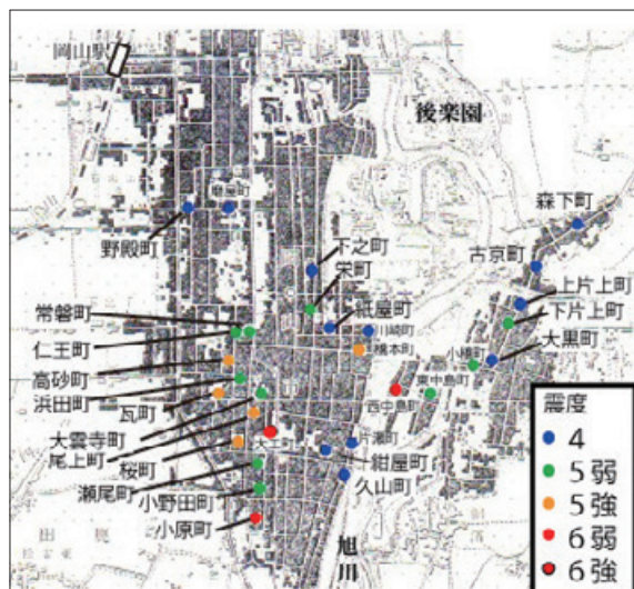
写真⑤ 安政南海地震による岡山城下 30 ケ町の震度分布
